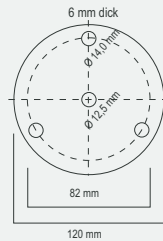
Fußplatte für Poller Ø 60 mm
