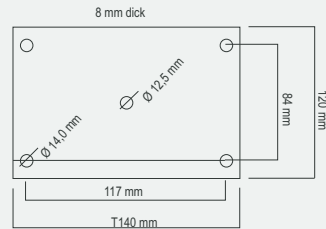
Fußplatte für Poller ab Ø 76 mm
