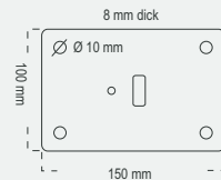
Fußplatte für klappbare Poller
