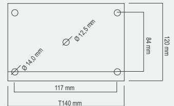
Fußplatte für Poller ab Ø 76 mm
