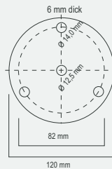
Fußplatte für Poller Ø 60 mm
